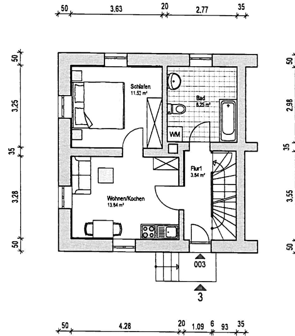
ERDGESCHOSS
