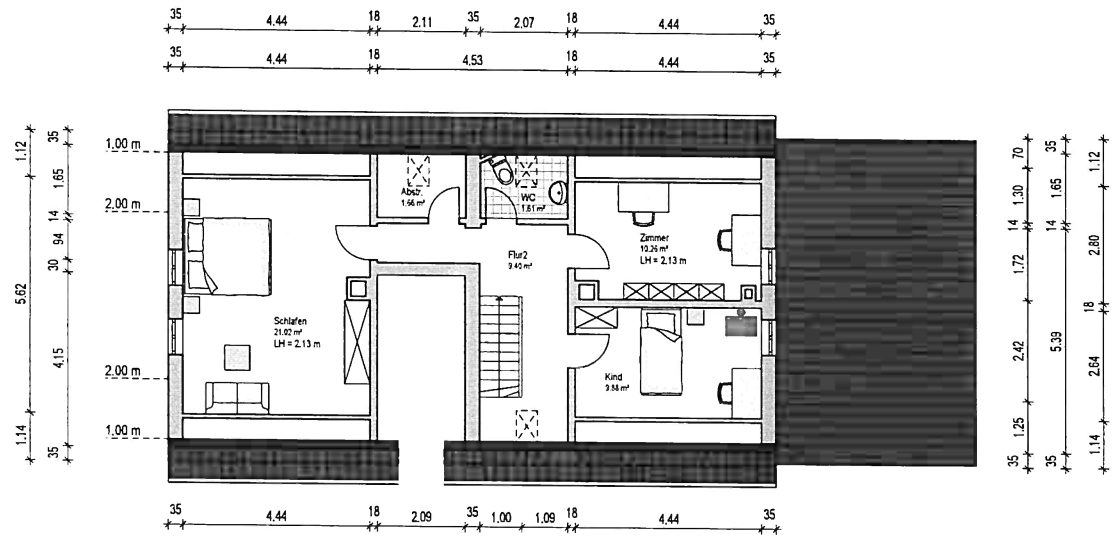
OBERGESCHOSS
