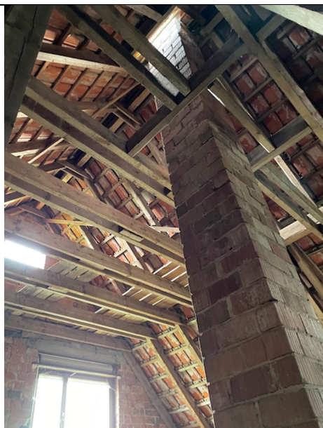
Dachkonstruktion
